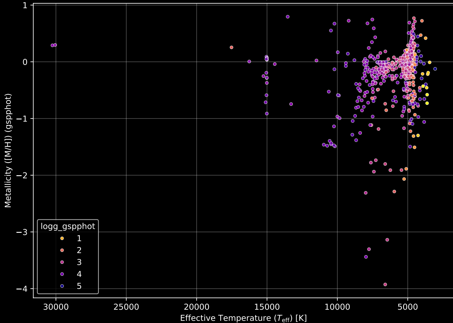
APOGEE DR17 Field: [090+00] Stellar Population Parameters (n= 706)
